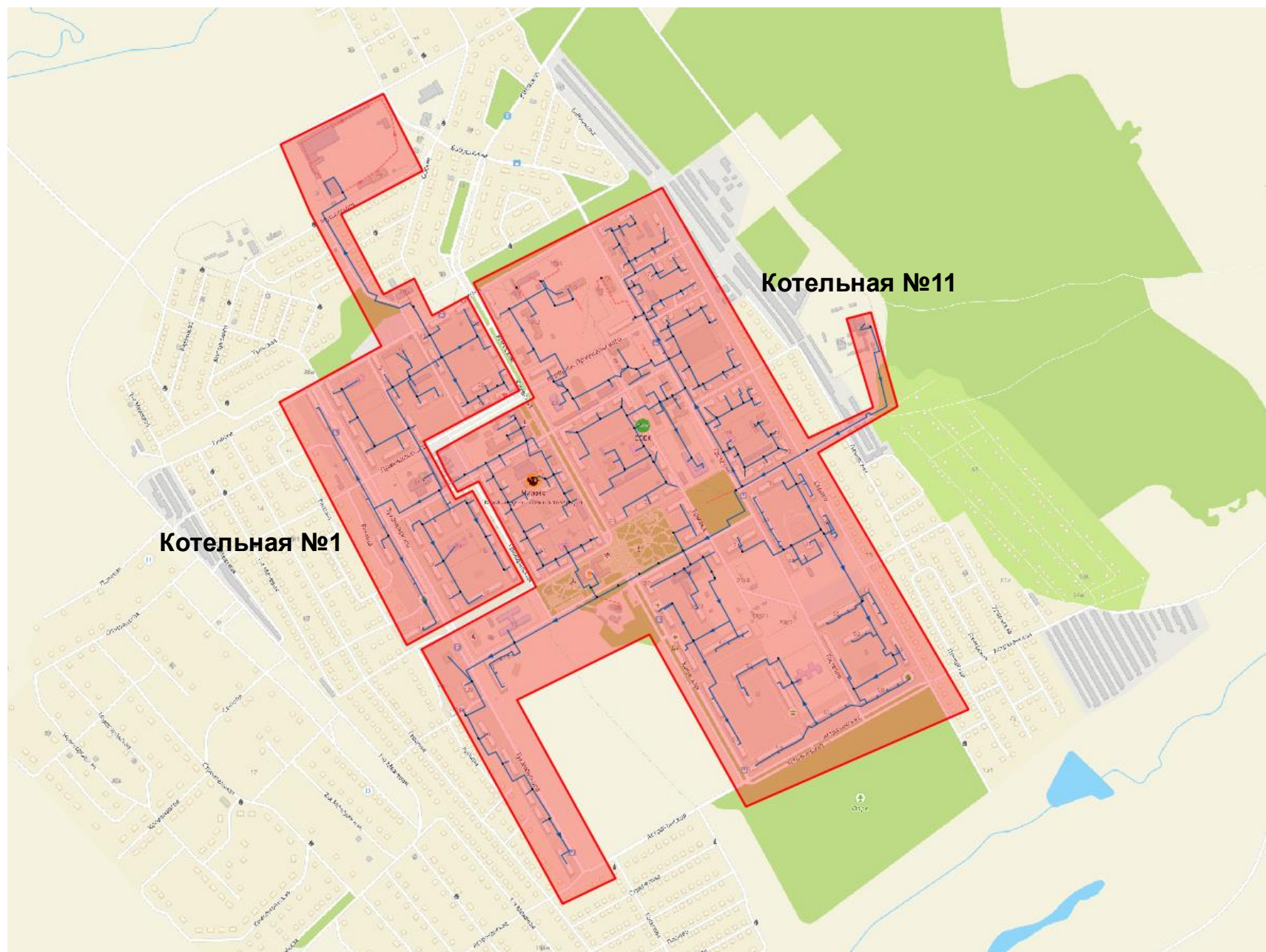
Рисунок 2.1 - Схемы тепловых сетей Котельной №1 и Котельной №11
