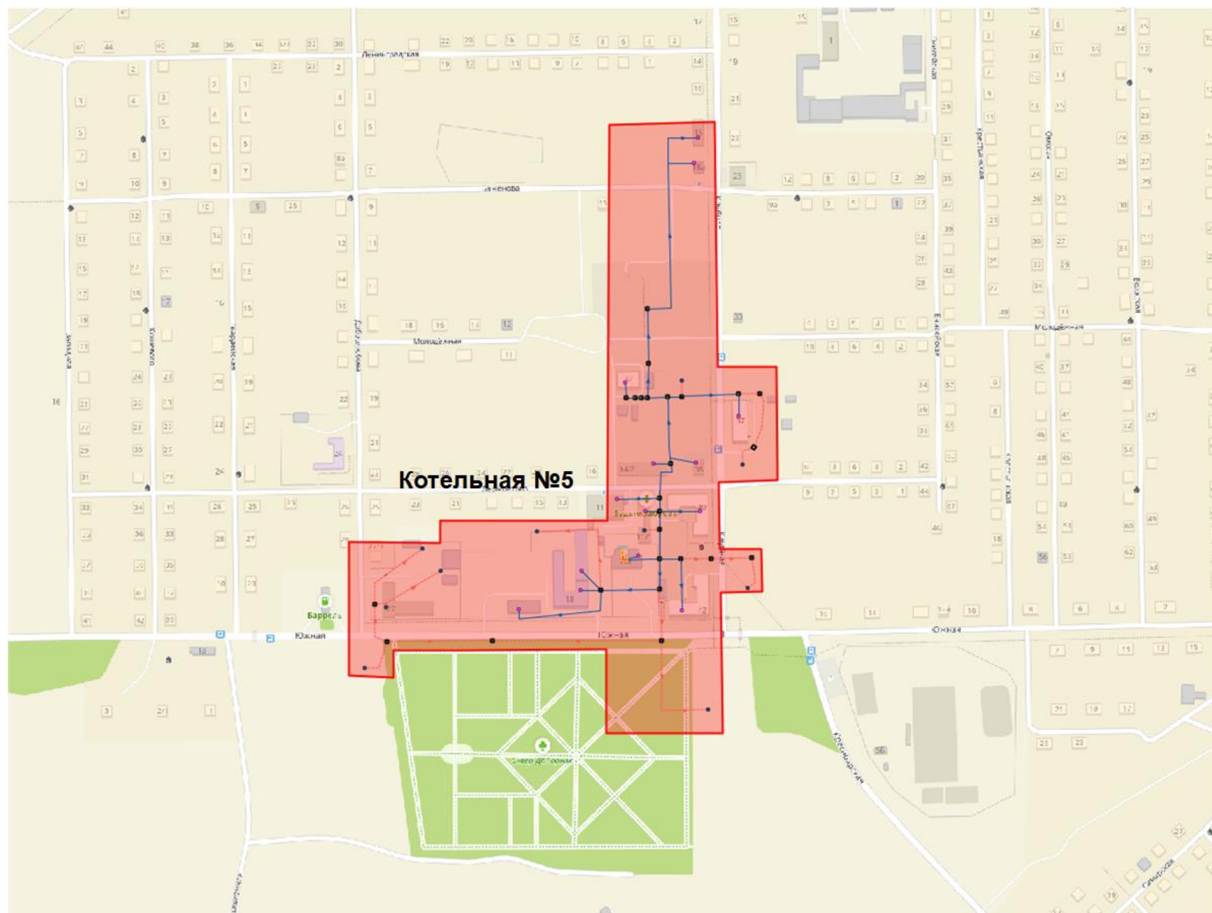
Рисунок 2.2 - Схемы тепловых сетей Котельной №5
