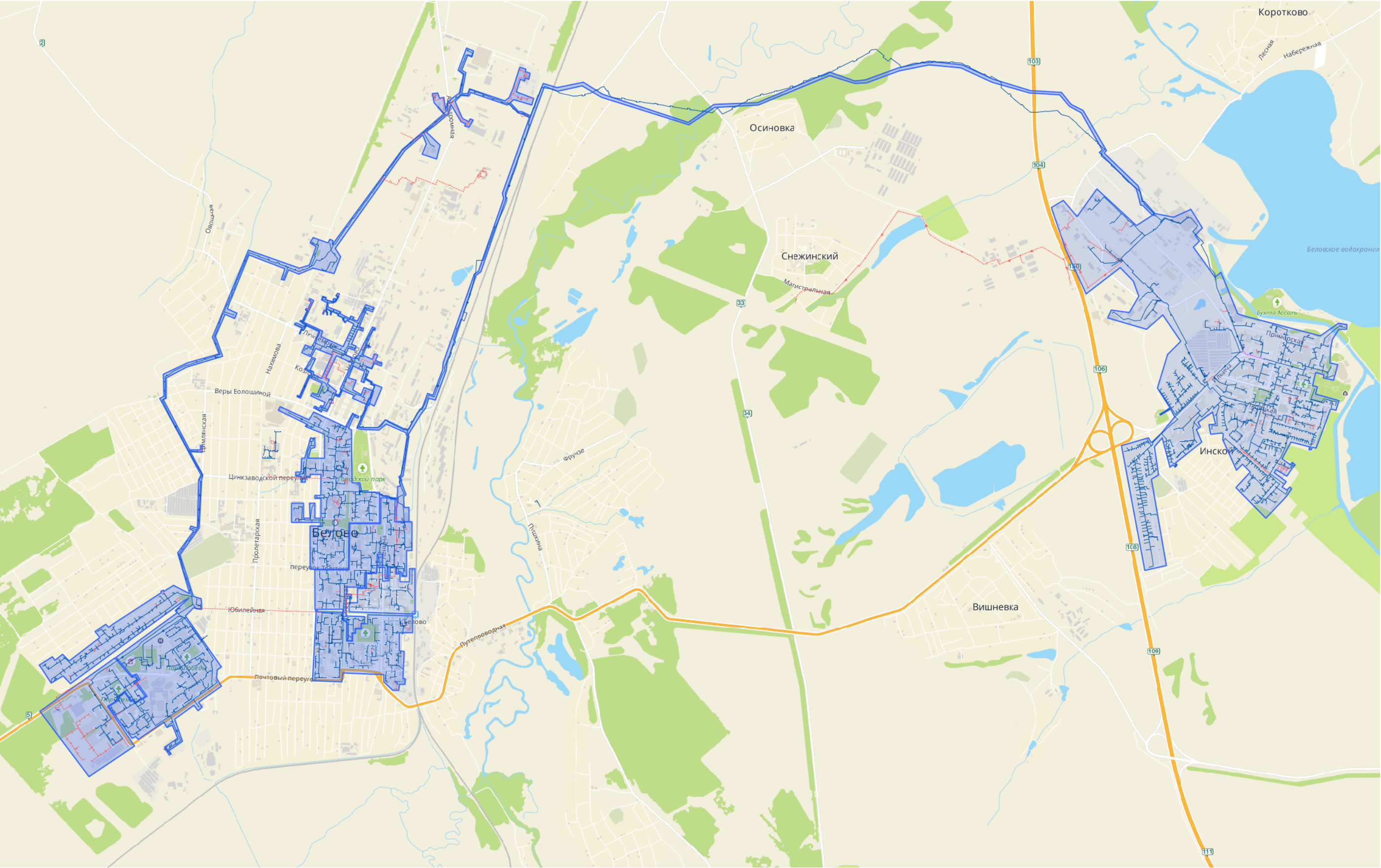
Рисунок 1.1 - Схема тепловых сетей Беловской ГРЭС
