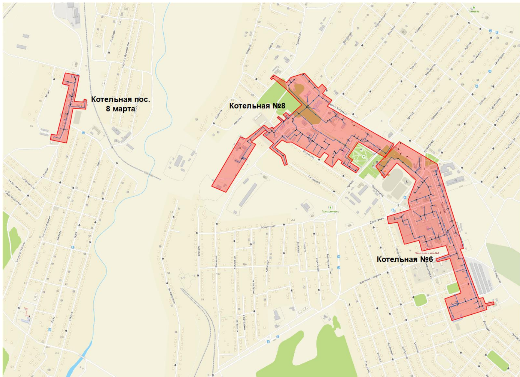
Рисунок 2.3 - Схемы тепловых сетей Котельной №6, Котельной №8 и Котельной пос. 8 марта
