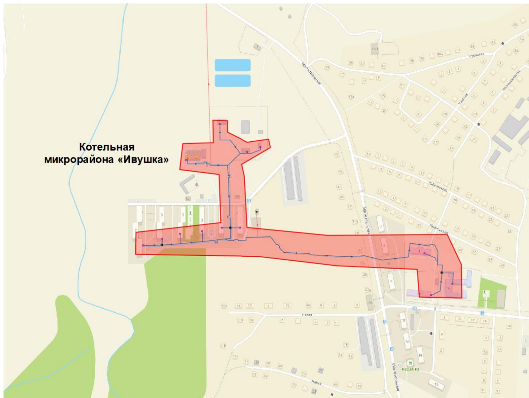
Рисунок 2.4 - Схема тепловых сетей Котельной микрорайона «Ивушка»
