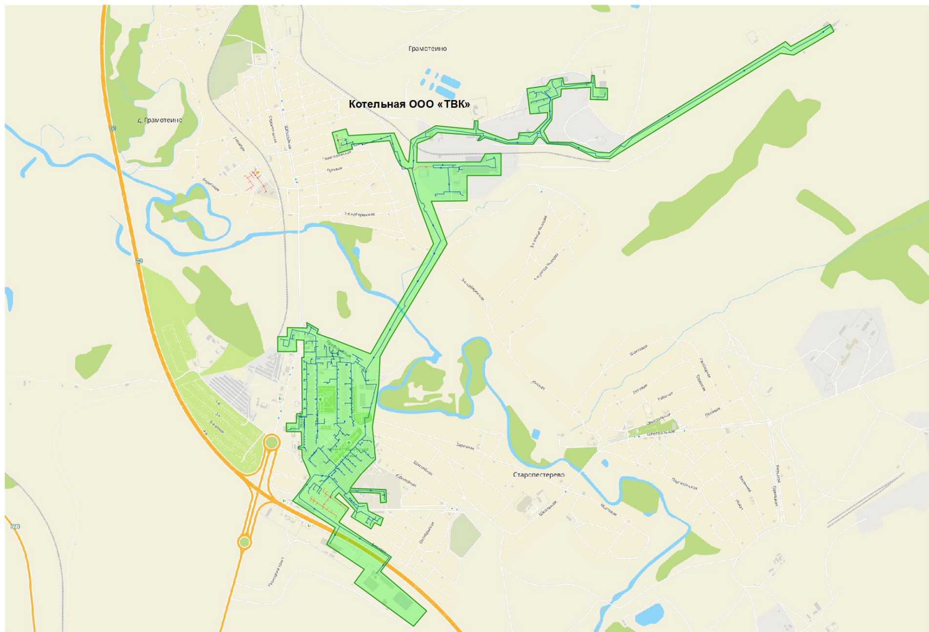
Рисунок 4.1 - Схема тепловых сетей Котельной ООО «ТБК»
