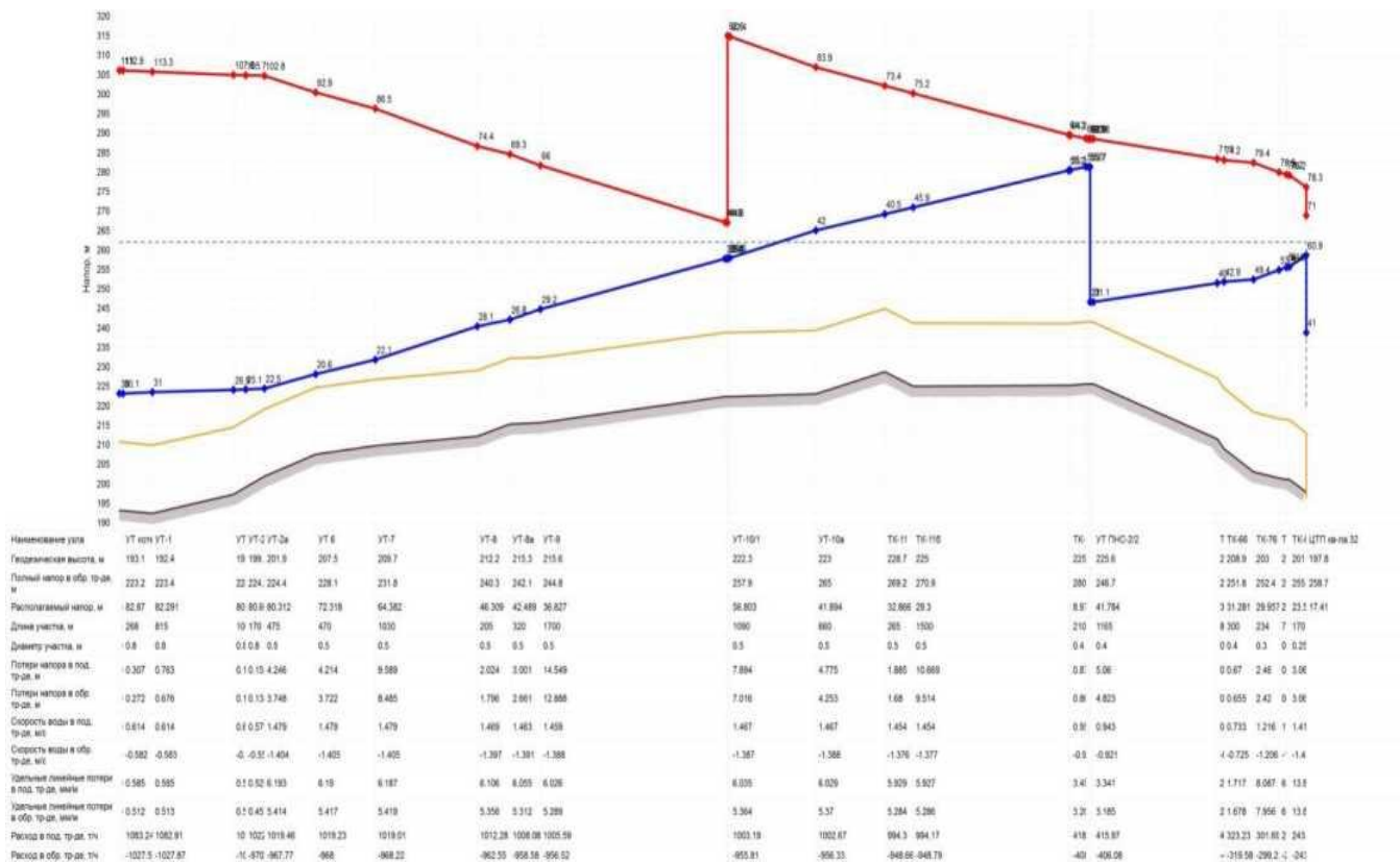
Рис. 3.4.12. Пьезометрический график
