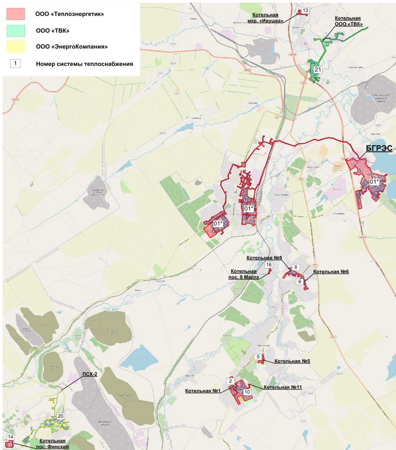
Рис. 6.1. Границы зон деятельности единых теплоснабжающих организаций Беловского городского округа при актуализации схемы теплоснабжения на 2026 год
