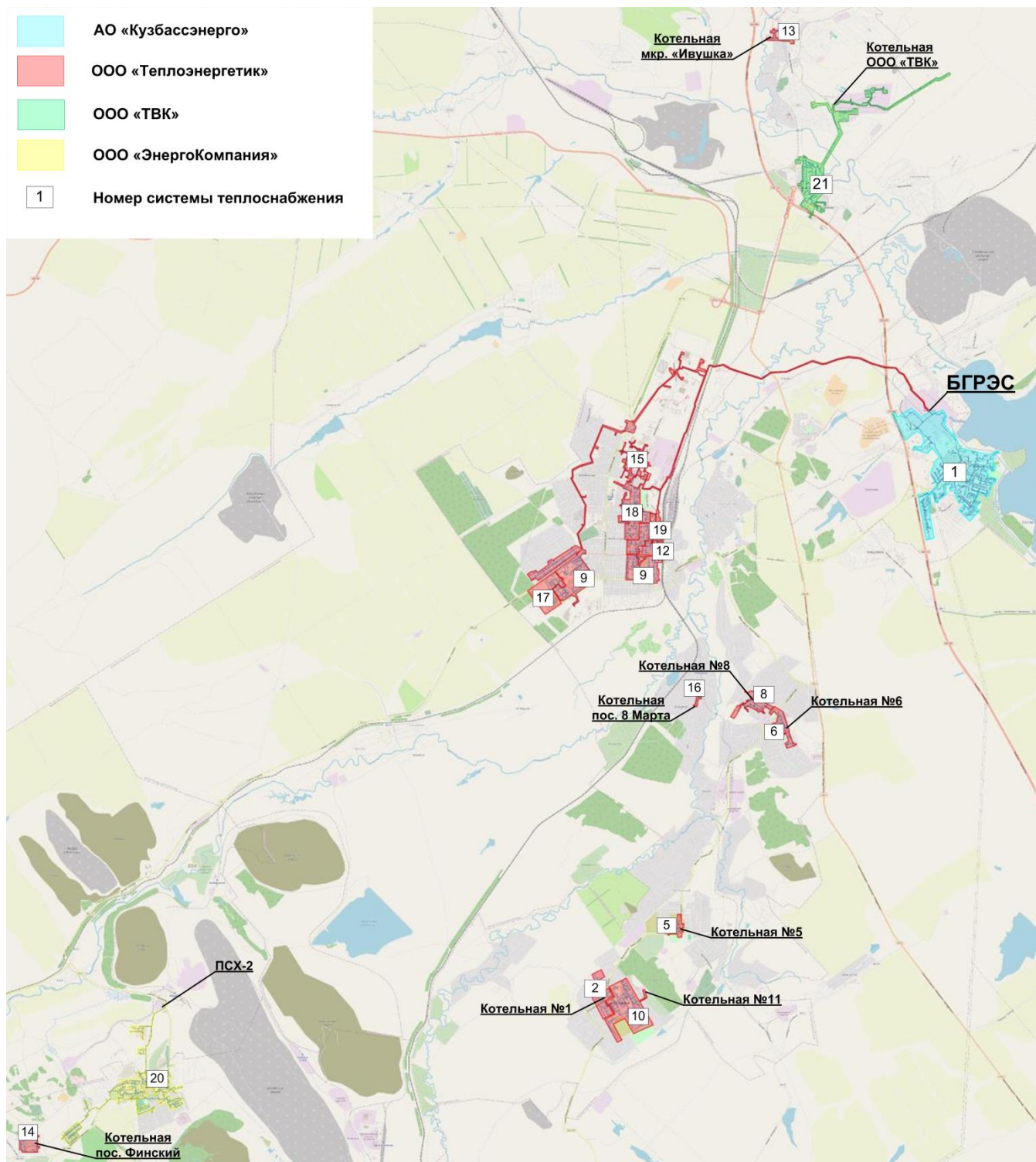
Рис. 5.1. Границы зон деятельности единых теплоснабжающих организаций Беловского городского округа
