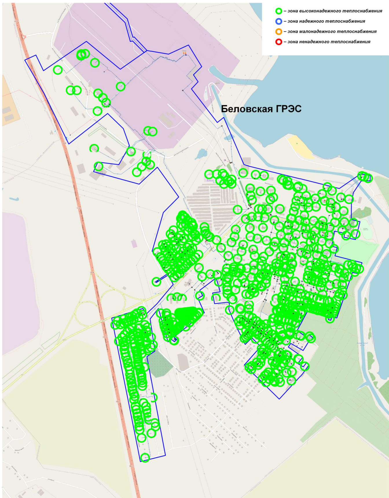
Рис. 9.4.2. Зоны ненормативной надежности и безопасности теплоснабжения пос. Инской
