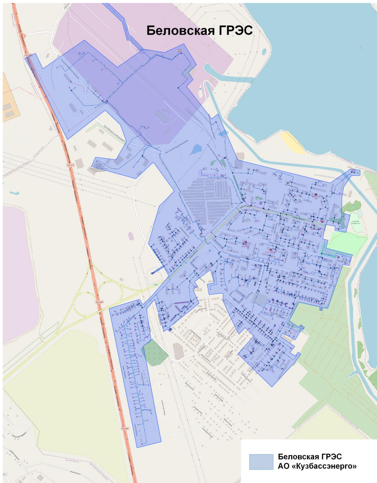
Рис. 4.1. Существующие зоны действия источников тепловой энергии в п. Инской
