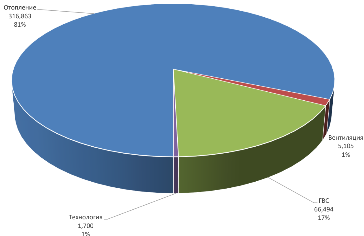
Рис. 1.2.2. Структура тепловой нагрузки в сетевой воде потребителей Беловского городского округа, подключенной к источникам теплоты Беловского городского округа
