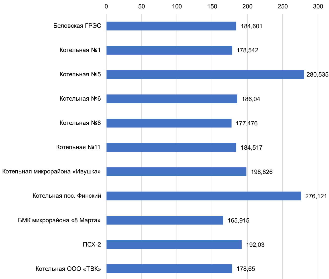
Рис. 8.1.1. Удельные расходы условного топлива на отпуск тепловой энергии источниками тепла системы теплоснабжения Беловского городского округа (кг у.т./Гкал)
