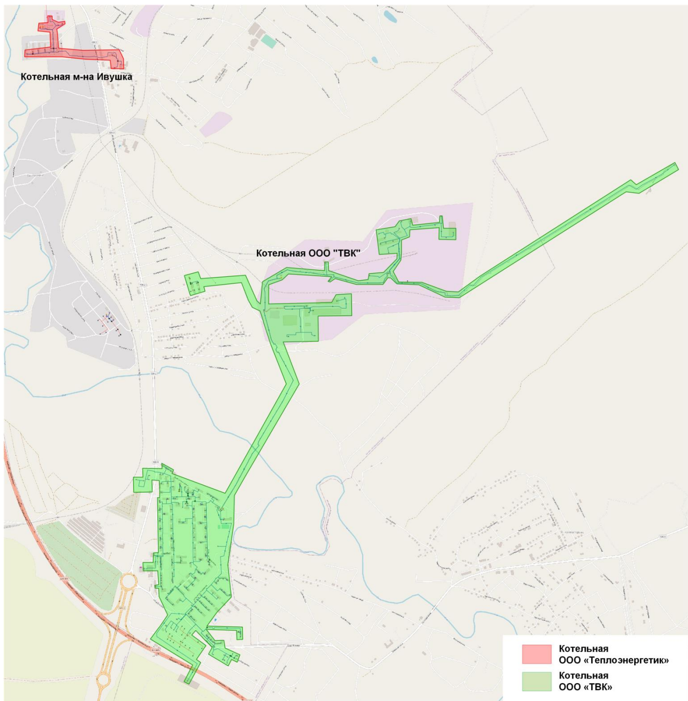
Рис. 4.4. Существующие зоны действия источников тепловой энергии в пгт. Грамотеино
