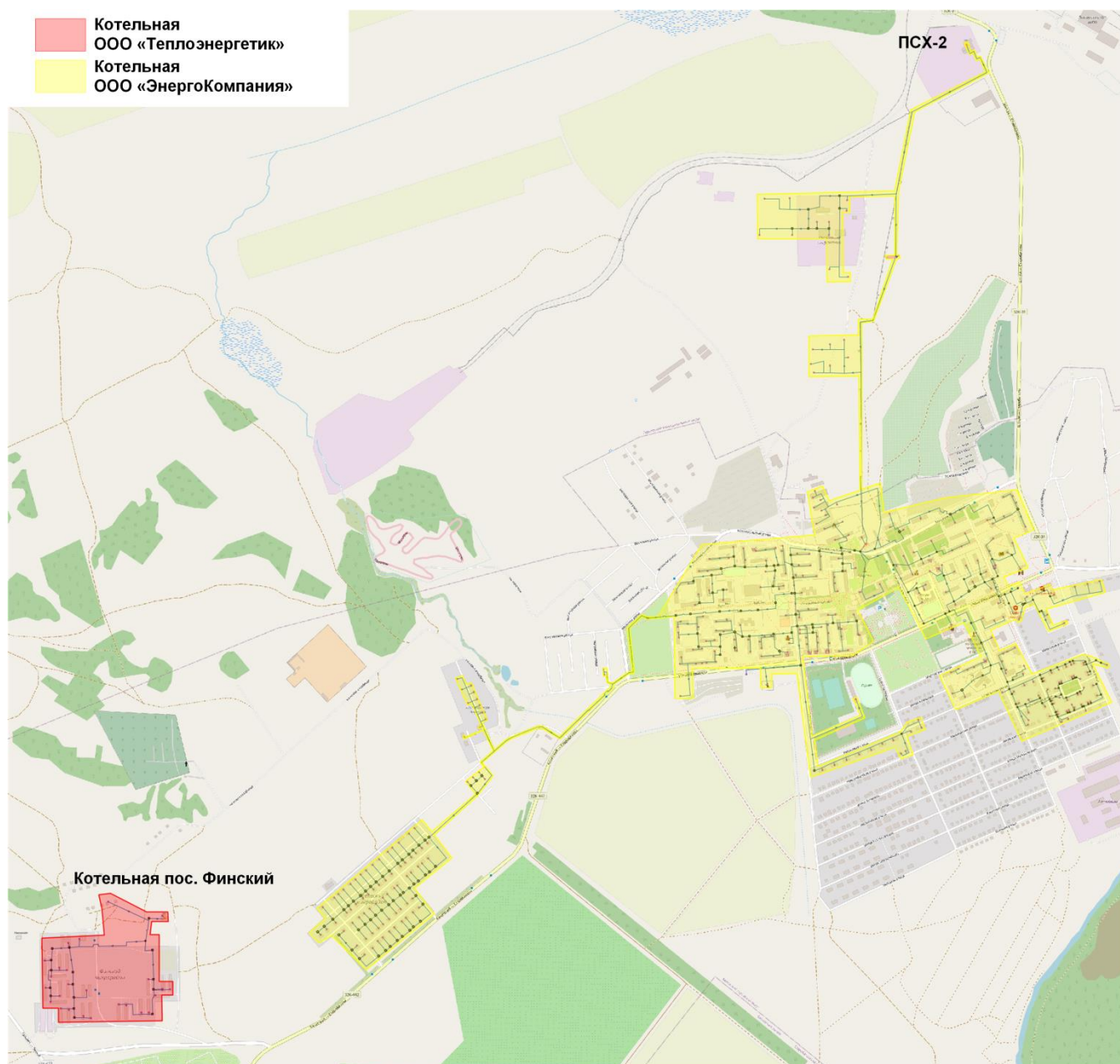
Рис. 4.5. Существующие зоны действия источников тепловой энергии в пгт Бачатский
