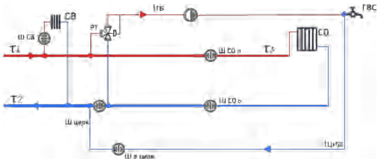
Рис. 1.2. Потребитель с открытым водоразбором на ГВС с циркуляцией и непосредственным присоединением СО
