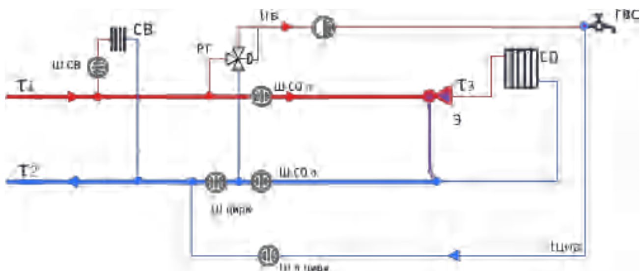
Рис. 1.4. Потребитель с открытым водоразбором на ГВС с циркуляцией и элеваторным присоединением СО
