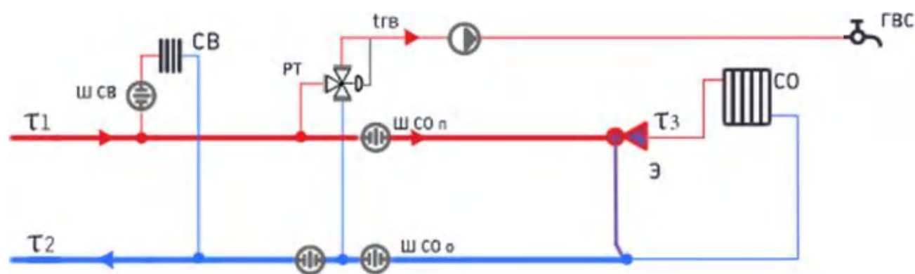
Рис. 1.3. Потребитель с открытым водоразбором на ГВС без циркуляции и элеваторным присоединением СО
