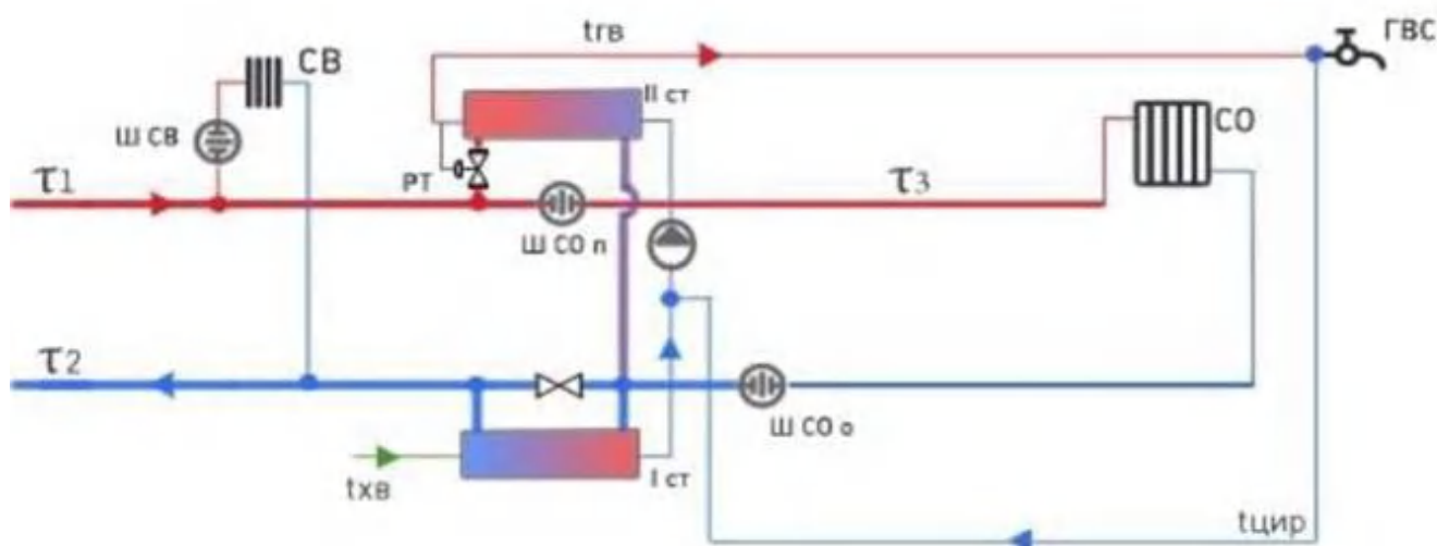
Рис. 1.6. Двухступенчатая (смешенная) схема присоединения подогревателей ГВС с зависимым присоединением системы отопления
