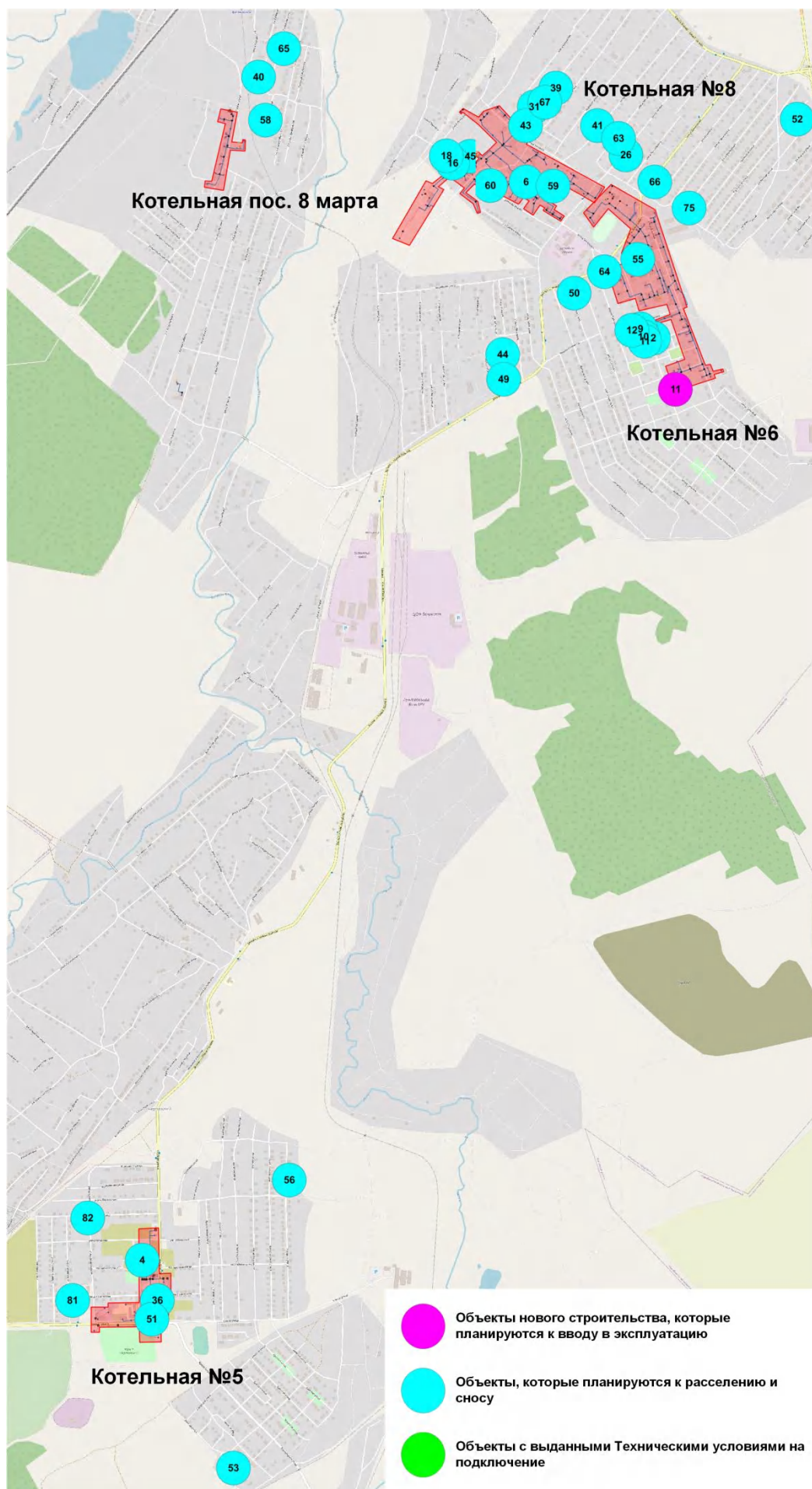
Рис. 1.1 Зоны действия источников теплоты г. Белово с перспективной застройкой
