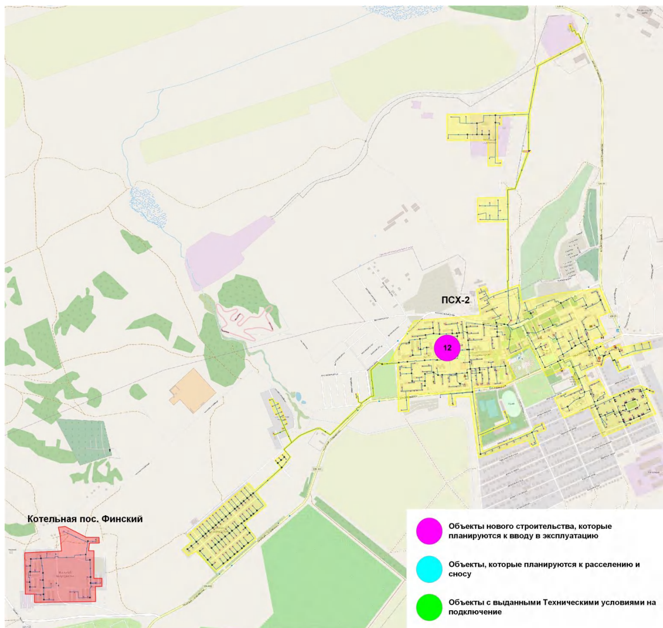
Рис. 1.5 Зоны действия источников теплоты пгт. Бачатский с перспективной застройкой
