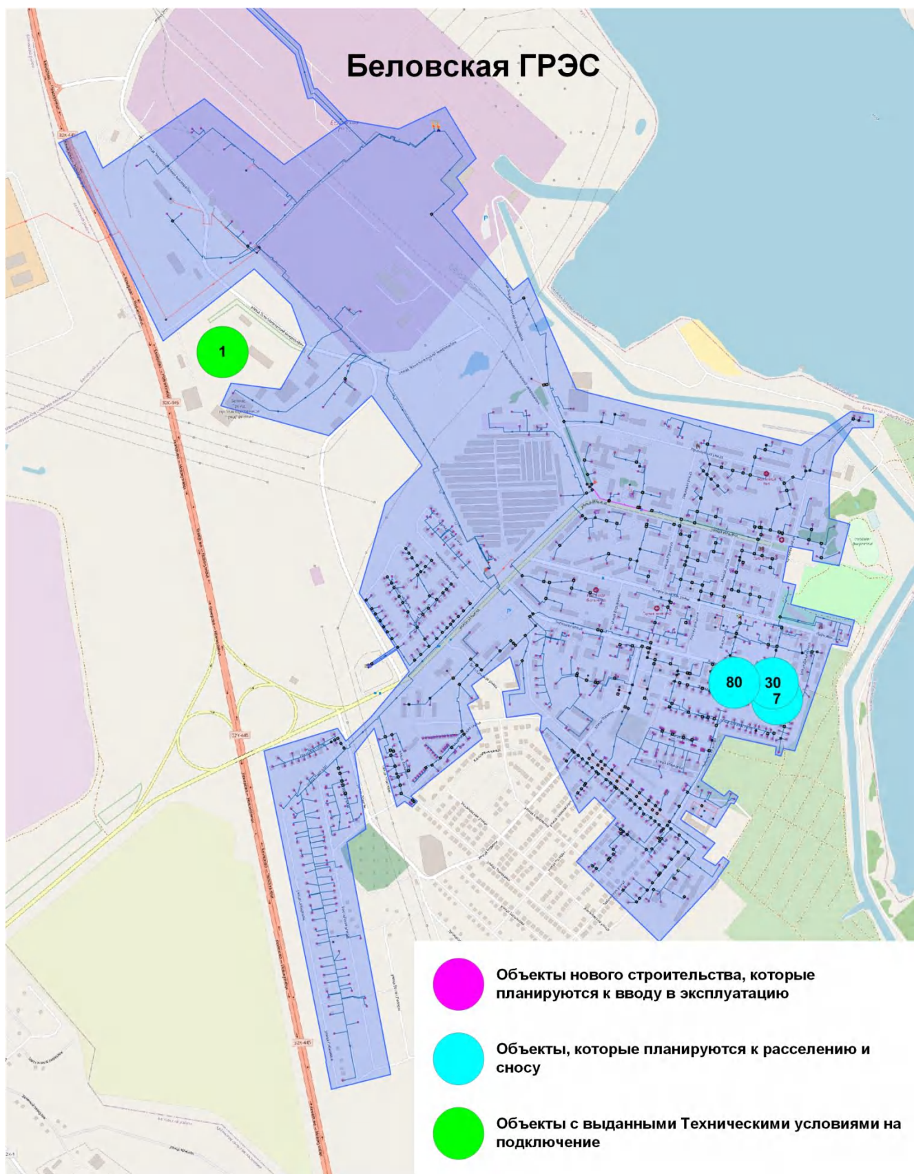
Рис. 1.2 Зоны действия источников теплоты п. Инской с перспективной застройкой
