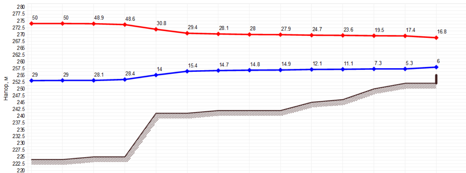
Пьезометрический график - от «Котельная №8» до «Больница №3, детск.отд.ул. Энп»
