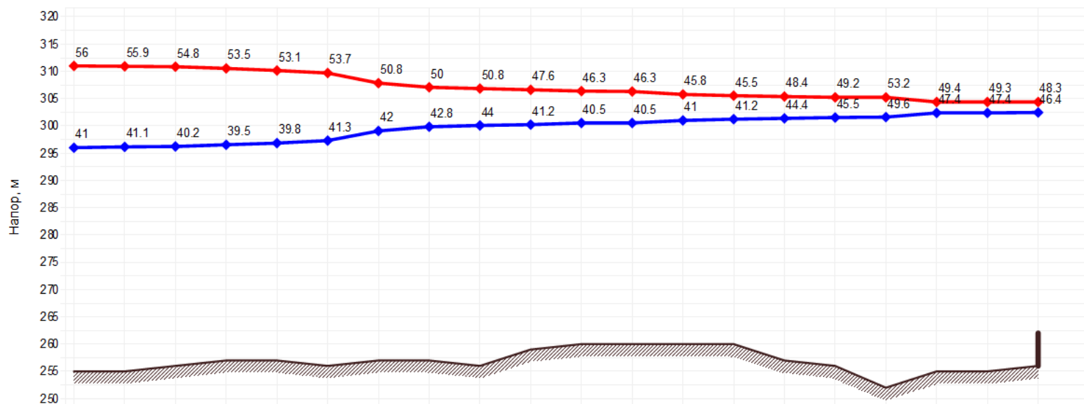
Пьезометрический график - от «Котельная №6» до «Стадион ул. Тимирязева, 32»
