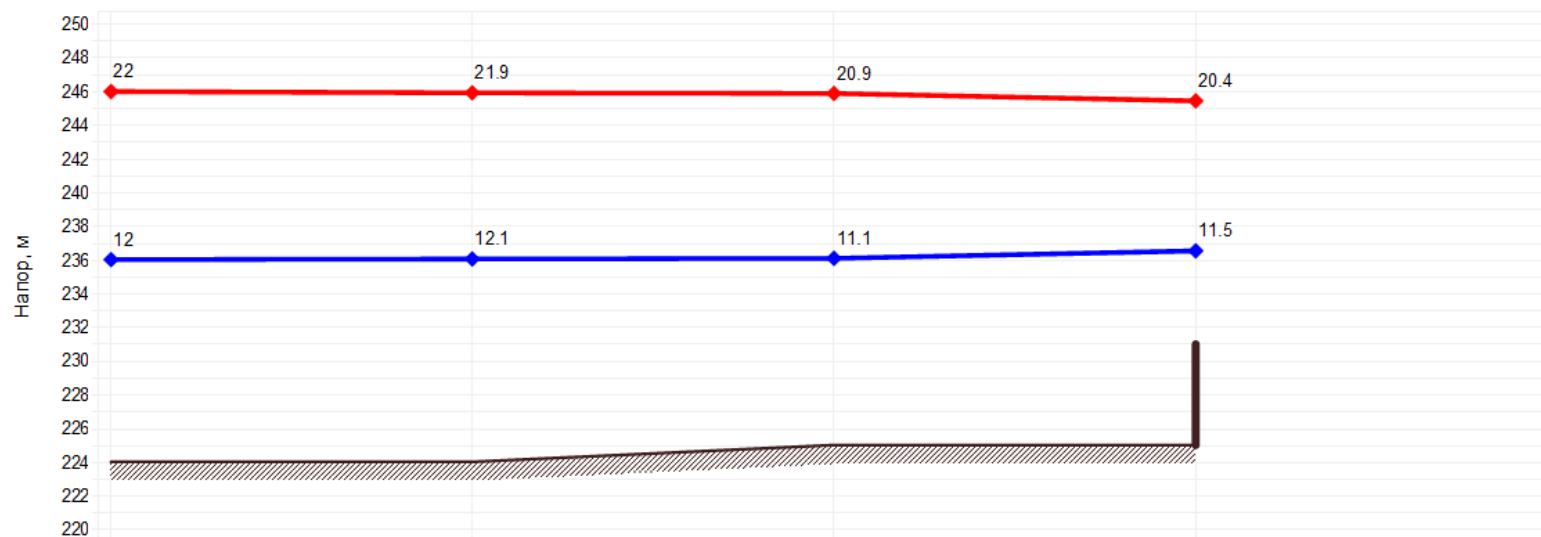
Пьезометрический график - от «Котельная №3» до «ж/д ул. Грамотеинская, 37»
