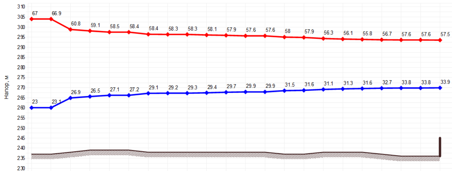
Пьезометрический график - от «Котельная №11» до «ж/д ул. Тухачевского, 22, ИП 3»
