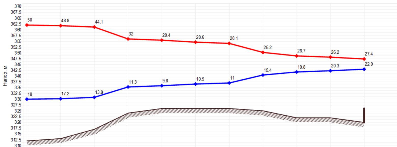
Пьезометрический график - от «Котельная пос. Финский» до «ж/д, Финский мкр-рн, 8»
