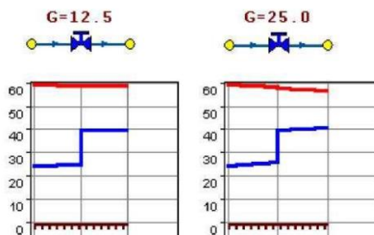
Рис. 3.4.11. Регулятор давления
