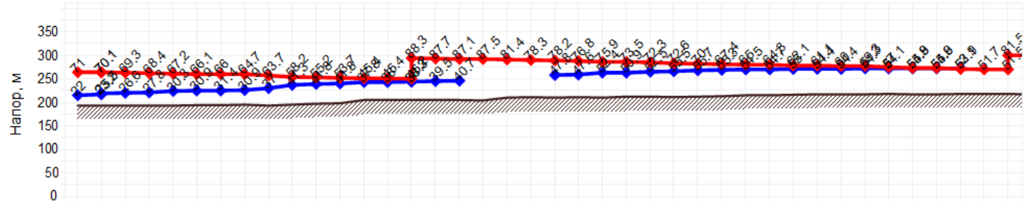
Пьезометрический график от «БГРЭС» до «жд ул. Дунаевского, 23»
