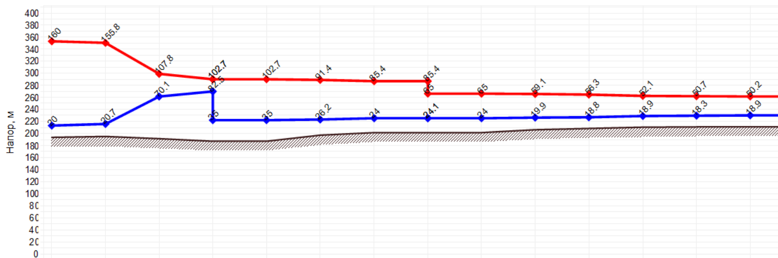
Пьезометрический график от «БГРЭС (т/м в г. Белово)» до «Школа №28, пер. Козлова, 2»
