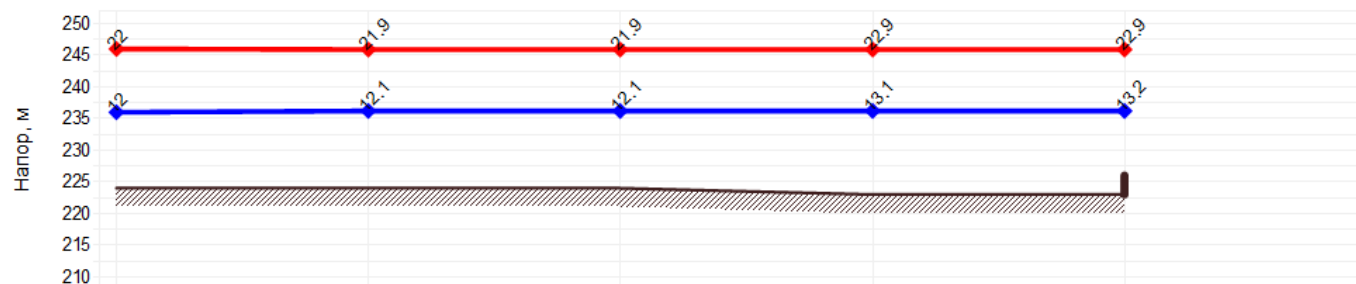
Пьезометрический график от «Котельная №3» до «Прачечная ул. Грамотеинская, 31»
