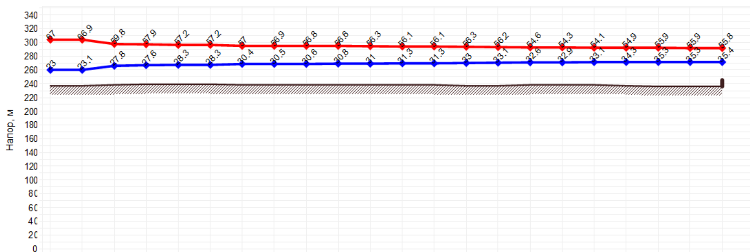
Пьезометрический график от «Котельная №11» до «ж/д ул. Тухачевского, 22, ИП 3»
