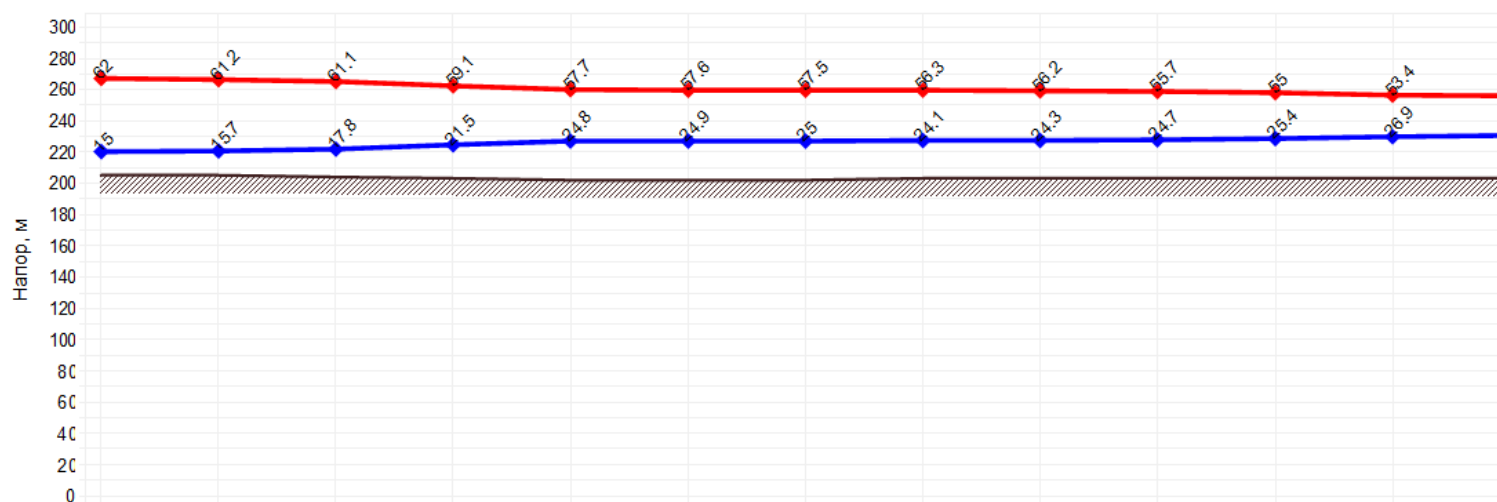
Пьезометрический график от «Котельная 30-го квартала(Сов.)» до «ФГУП Баланс, пер. Толстого, 18»
