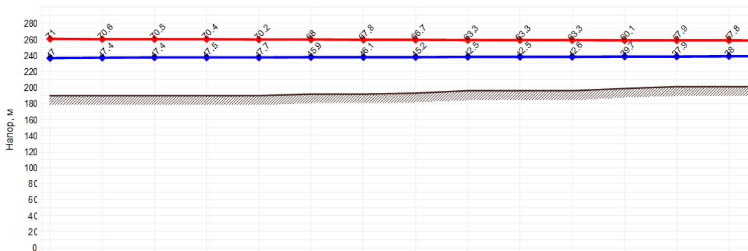
Пьезометрический график от «Котельная 34-го квартала» до «ж/д ул. Советская, 55»
