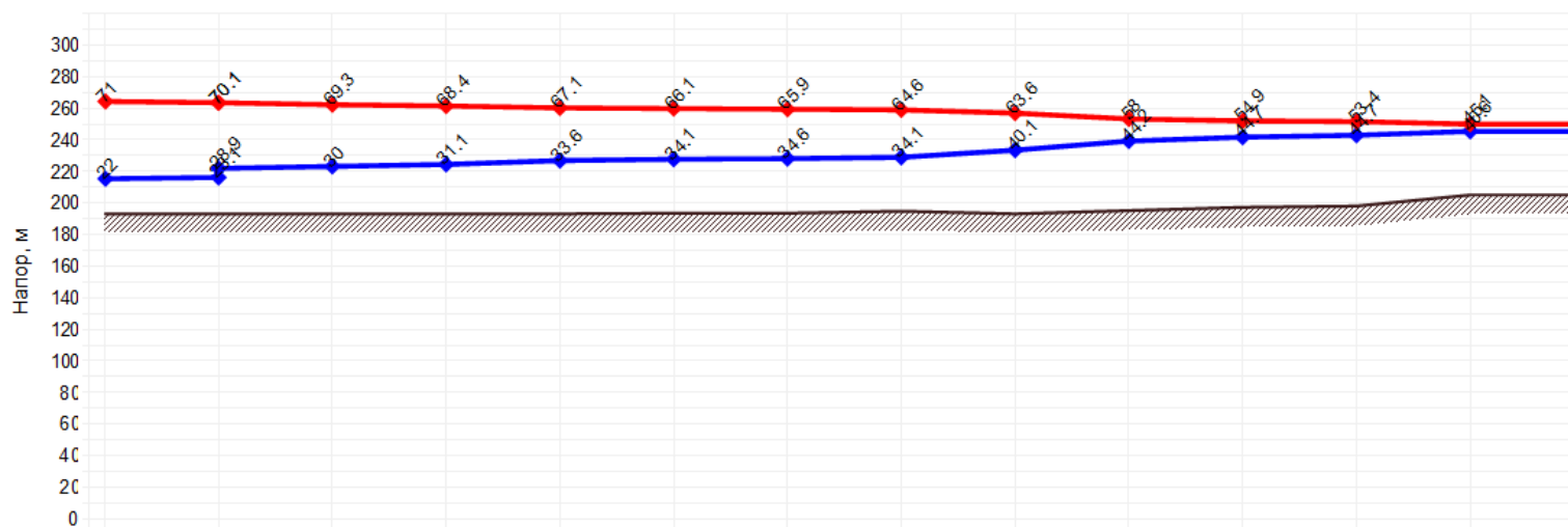
Пьезометрический график от «БГРЭС» до «МАУ ФОРЦ»
