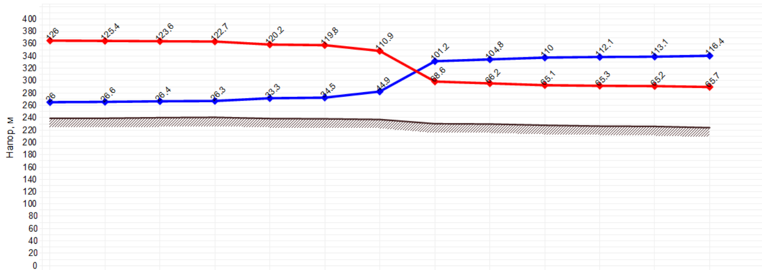
Пьезометрический график от «Кот. мкр. Сосновый» до «ж/д квартал Сосновый, 20/2»
