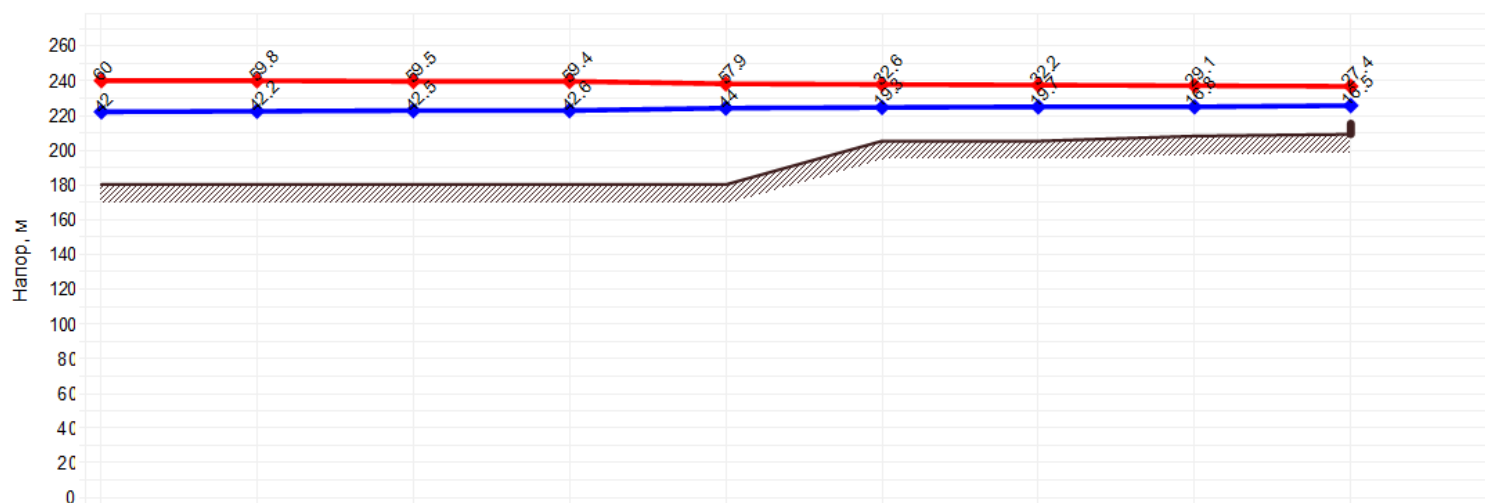
Пьезометрический график от «Котельная м-на Ивушка (от)» до «Д/сад №31 Лесная, 1в»
