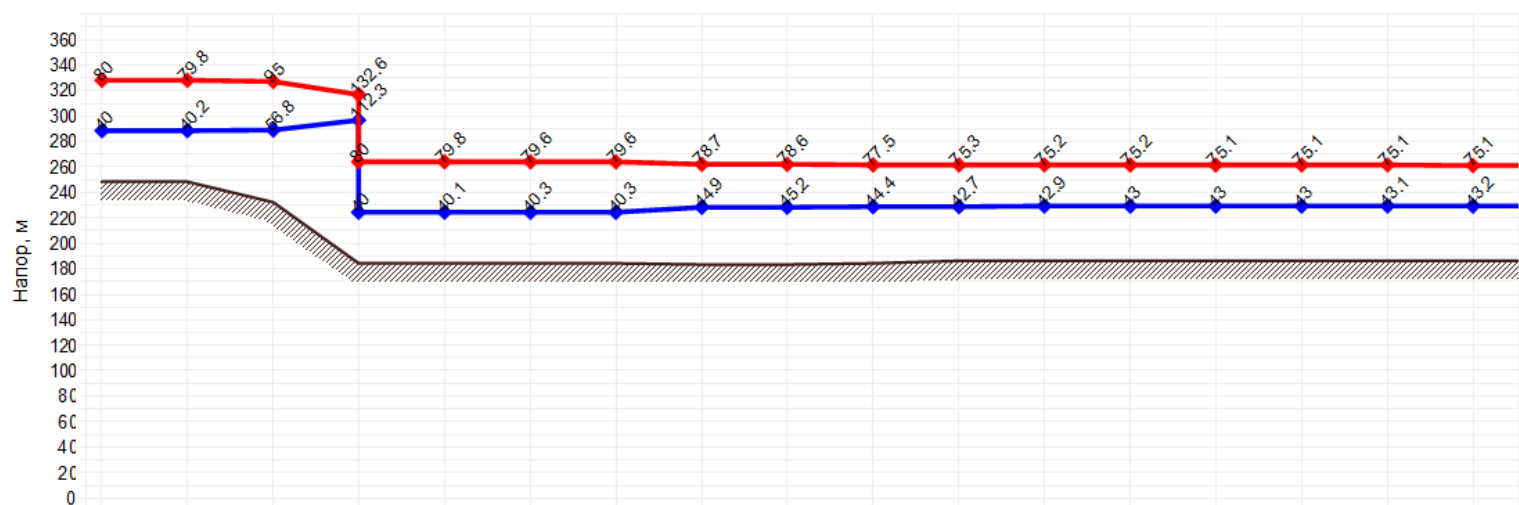
Пьезометрический график от «Котельная ООО "ТВК"» до «ж/д ул. Ворошилова, 20»
