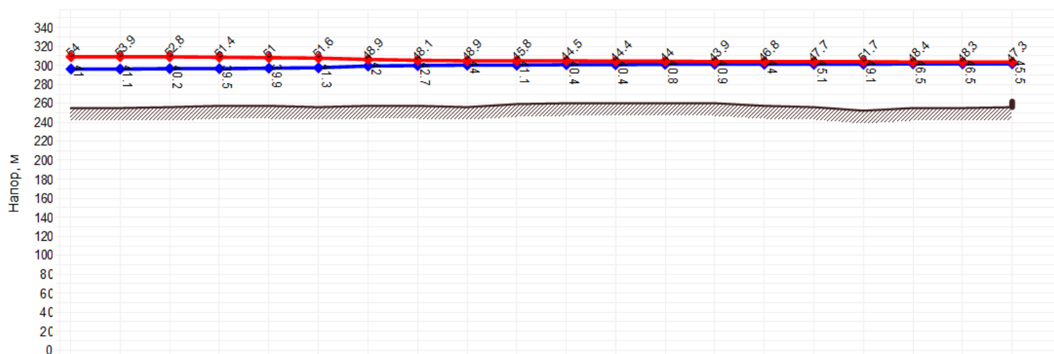
Пьезометрический график от «Котельная №6» до «Стадион ул. Тимирязева, 32»
