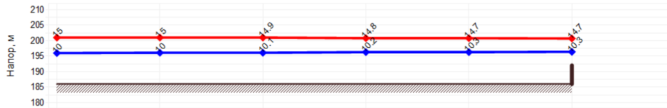
Пьезометрический график от «Котельная №2» до «ДЮСШ №2 ул. 7-е Ноября, 16»
