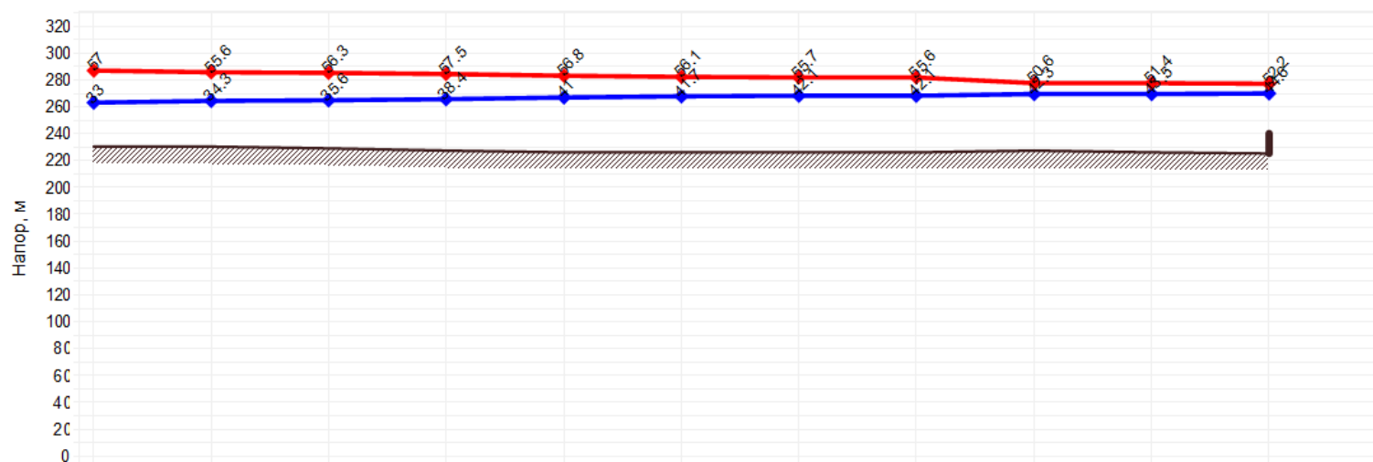
Пьезометрический график от «Котельная №1» до «ж/д ул. Глинки, 3»
