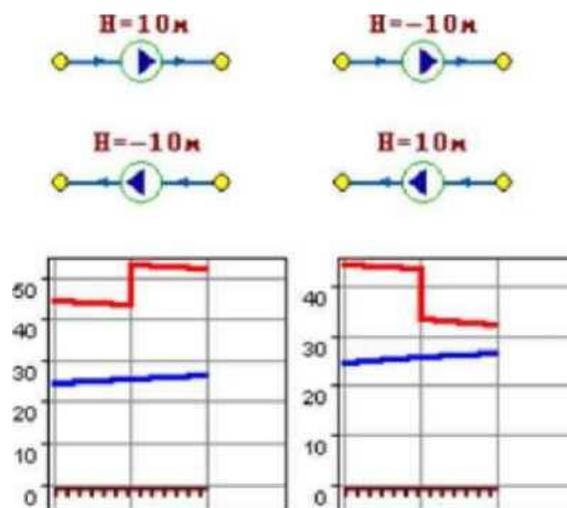
Рис. 3.4.7. Пьезометрические графики
