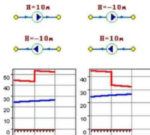
Рис. 3.4.7. Пьезометрические графики
