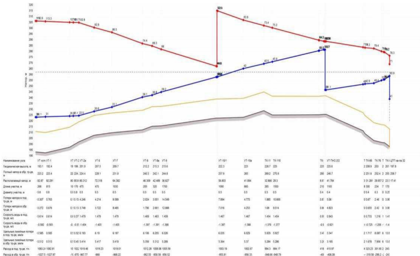
Рис. 3.4.12. Пьезометрический график
