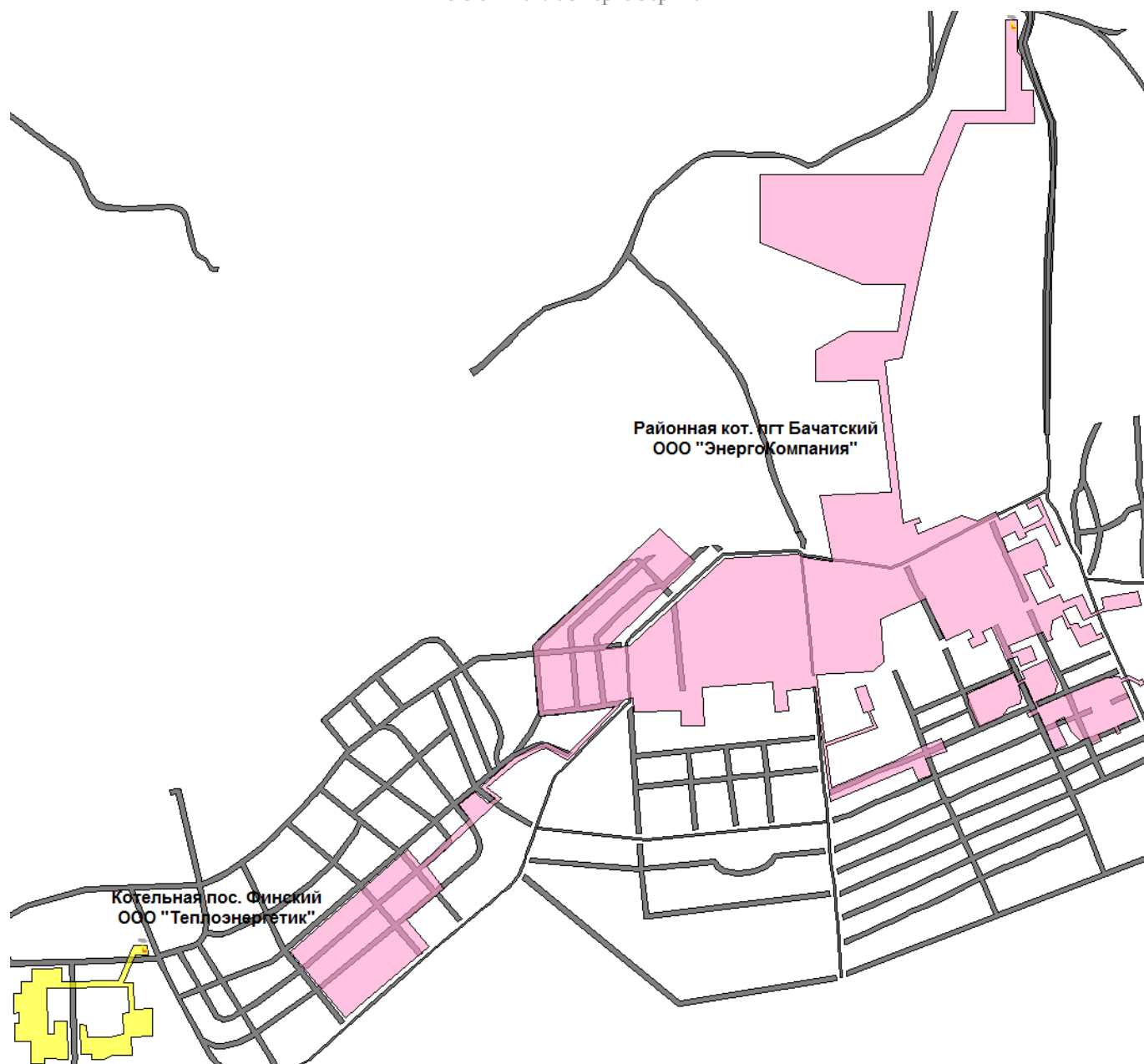
Рис. 2.12. Перспективные зоны действия тепловых источников в районе пгт. Бачатский по состоянию на 2028 г.
