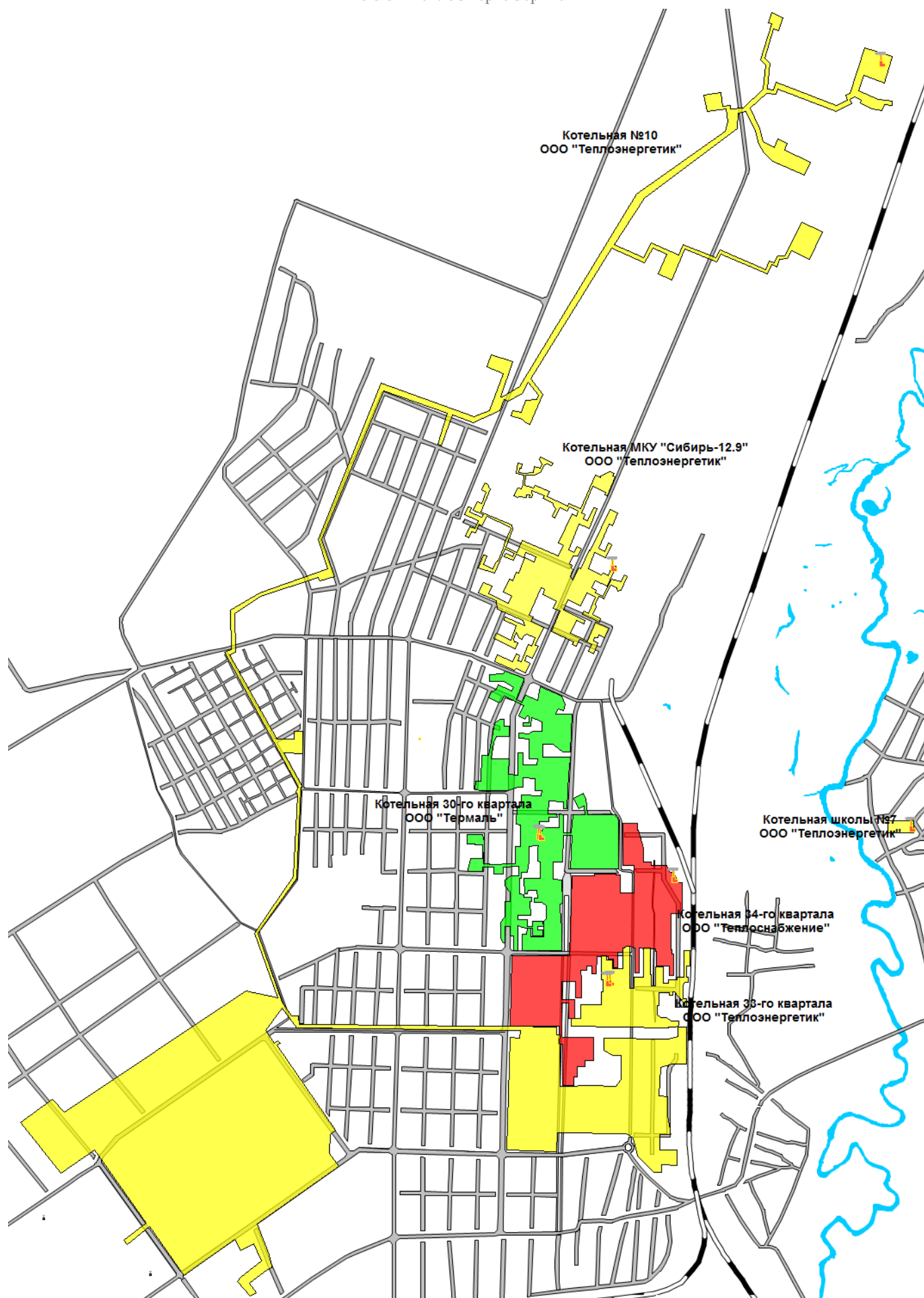
Рис. 2.2. Существующие зоны действия тепловых источников в Центральной части по состоянию на 2018 г. (начало)
