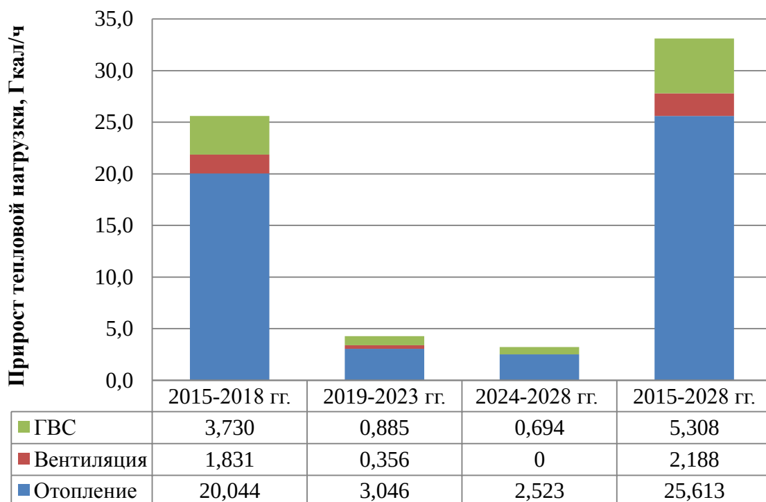
Рис. 1.8. Структура прогнозируемого прироста тепловой нагрузки перспективной застройки
