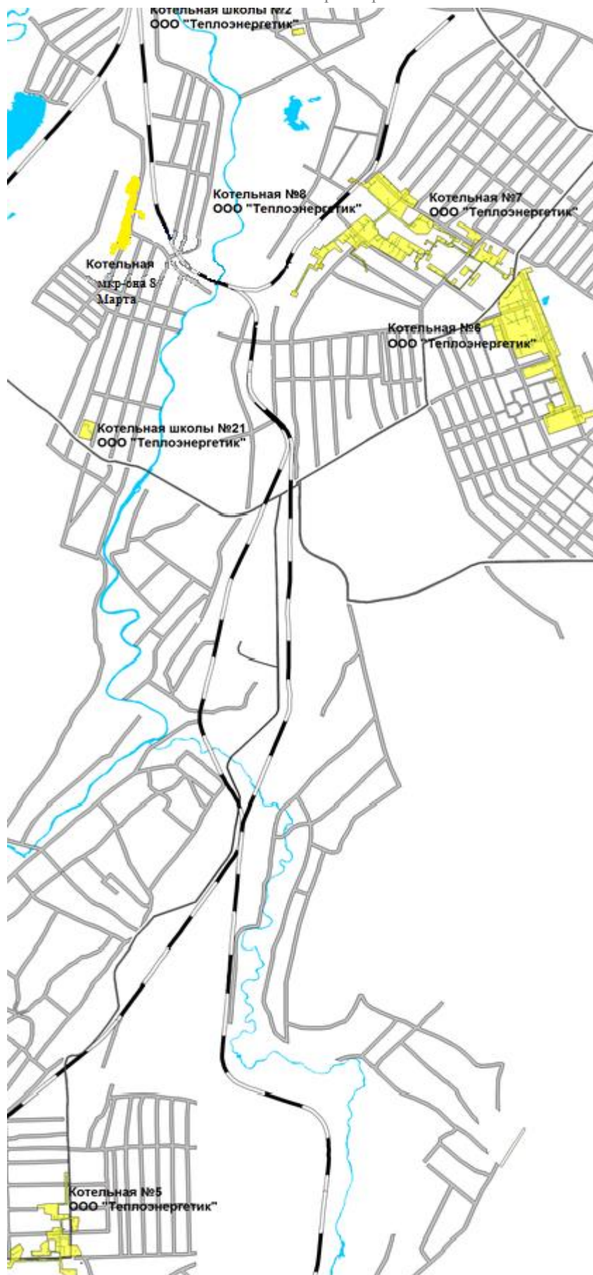
Рис. 2.3. Существующие зоны действия тепловых источников в Центральной части по состоянию на 2018 г. (окончание)
