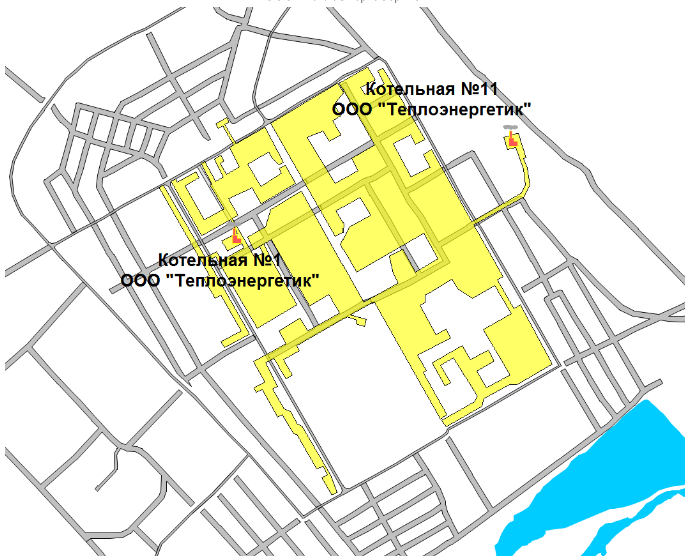
Рис. 2.5. Существующие зоны действия тепловых источников в районе пгт. Новый городок по состоянию на 2015 г.
