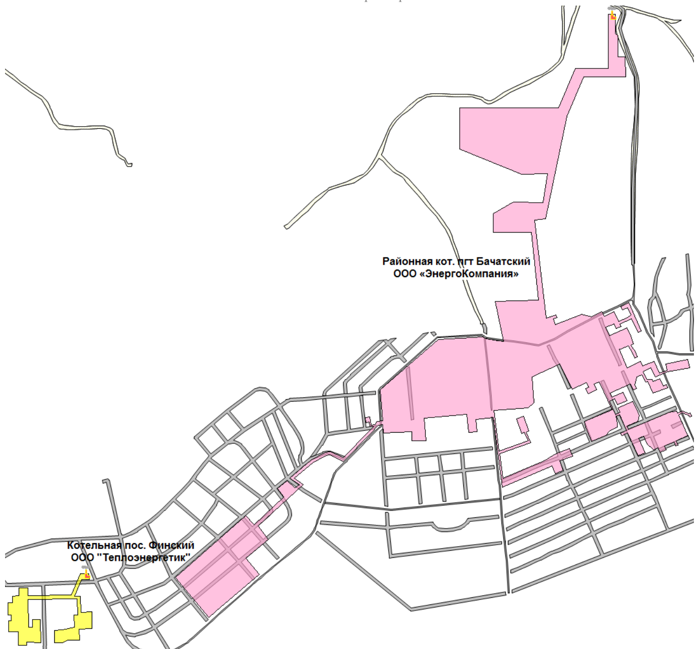
Рис. 2.6. Существующие зоны действия тепловых источников в районе пгт. Бачатский по состоянию на 2015 г.
