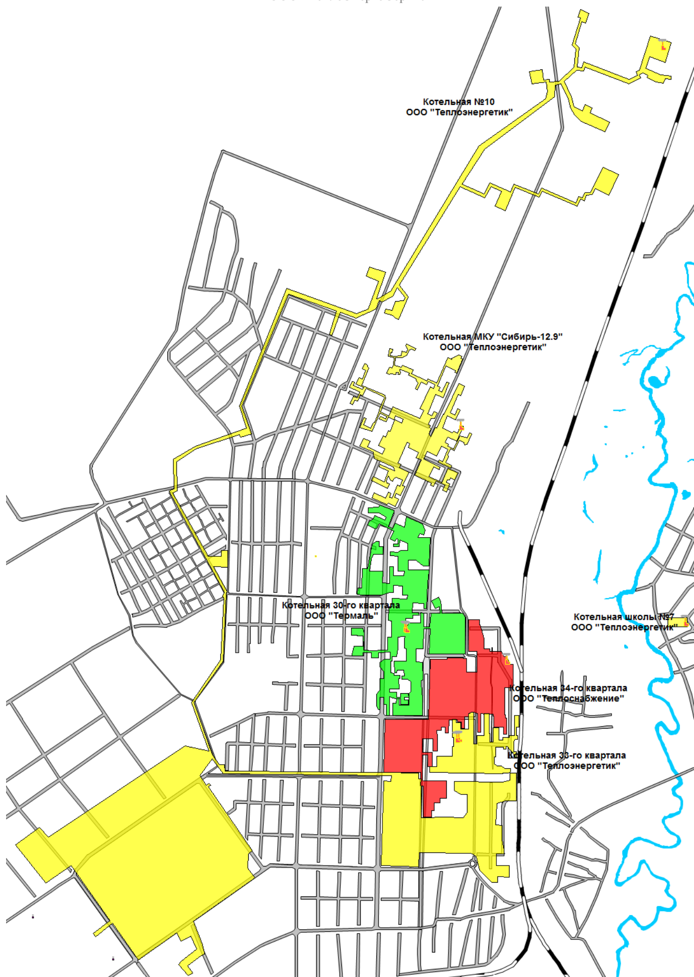
Рис. 2.2. Существующие зоны действия тепловых источников в Центральной части по состоянию на 2015 г. (начало)
